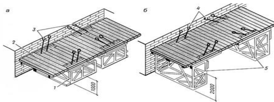
Рисунок 4.4 – Установка підмостків: а) для мурування 2-го ярусу; б) для мурування 3-го ярусу; 1 – прямокутні опори в нижньому положенні; 2 – робочий настил; 3 и 4 – стропи для переводу опор в вертикальне і горизонтальне положення; 5 – прямокутні опори ( studizba.com ) в вертикальному положенні.
