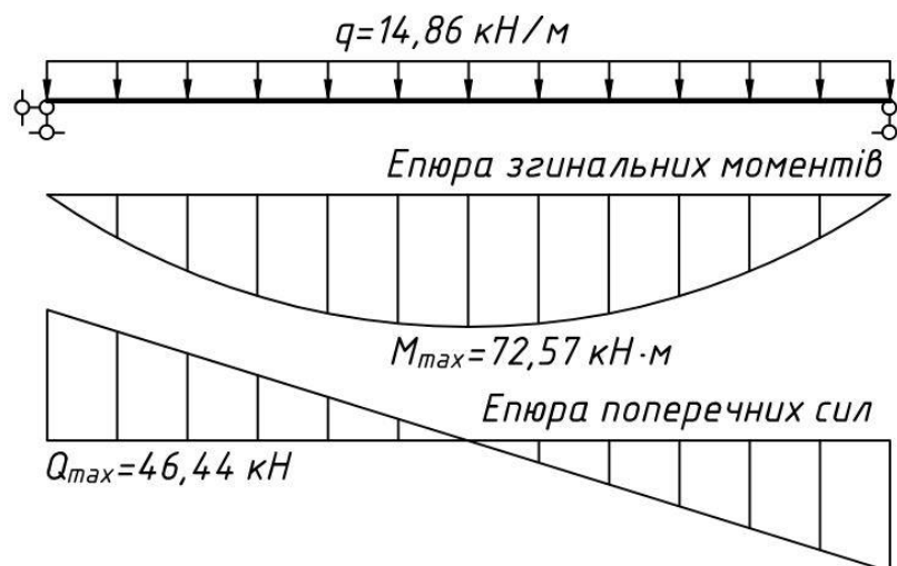
Рисунок 2.2 – Розрахункова схема балки,
