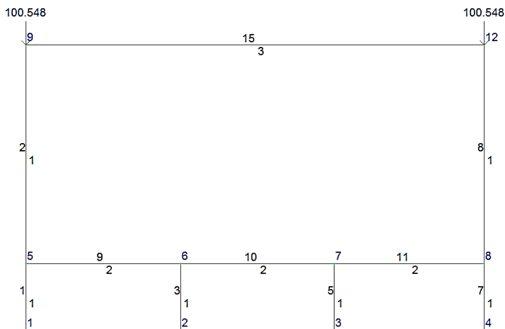
Рисунок 2.4 – Навантаження №3 - снігове
