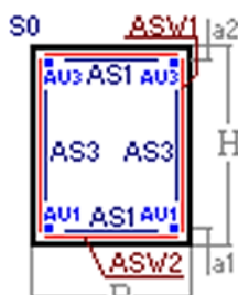
Рисунок 2.6 – Схема розташування арматури
