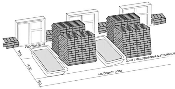
Рисунок 4.1 – Організація робочого місця для стін: а) глухих, б) простінків
