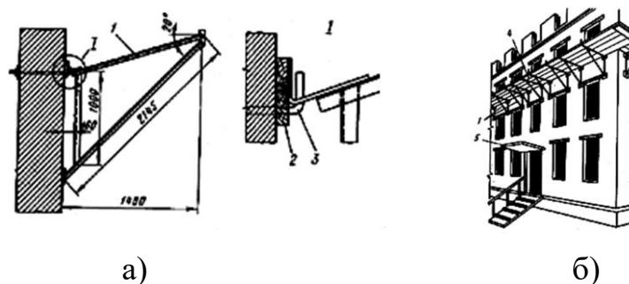
Рисунок 4.3 – Захисні козирки
