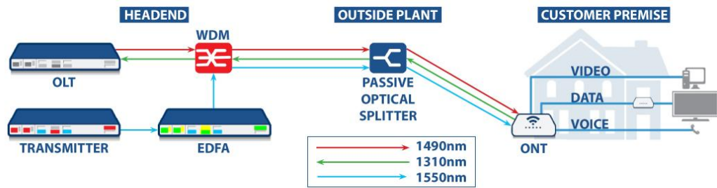
Рисунок 2.2 - Типова мережа GPON з радіочастотним покриттям
