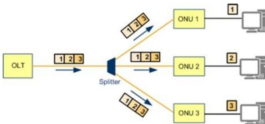
Рисунок 2.8 – Схема шляху пакетів до користувачів
