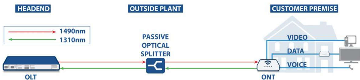
Рисунок 2.4 – Схема GPON OLT
