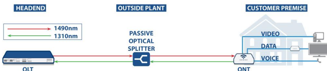
Рисунок 2.1 - Типова мережа GPON
